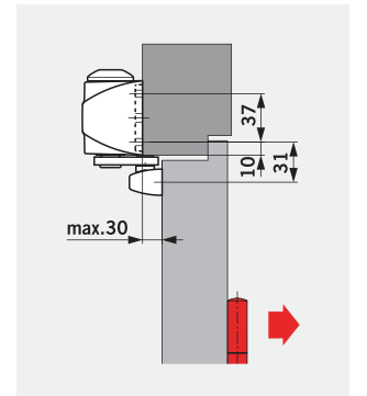
Kapı kasasına itme yönünde montaj
